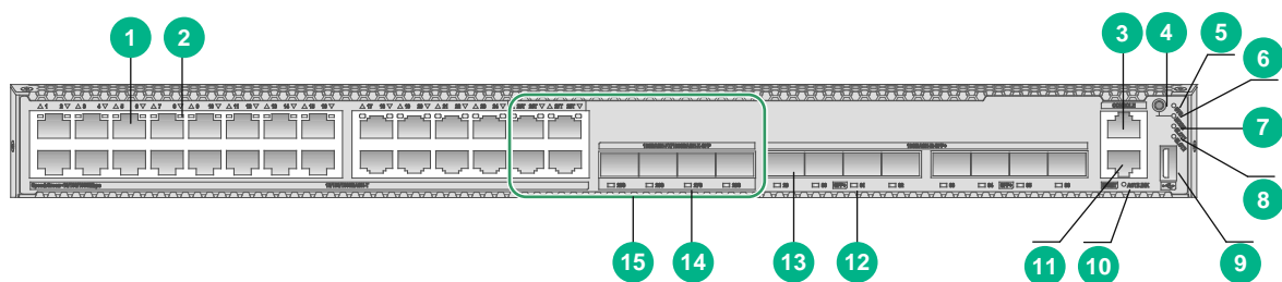
图2-1 S5800XP-40C-HI-G 前面板示意图
