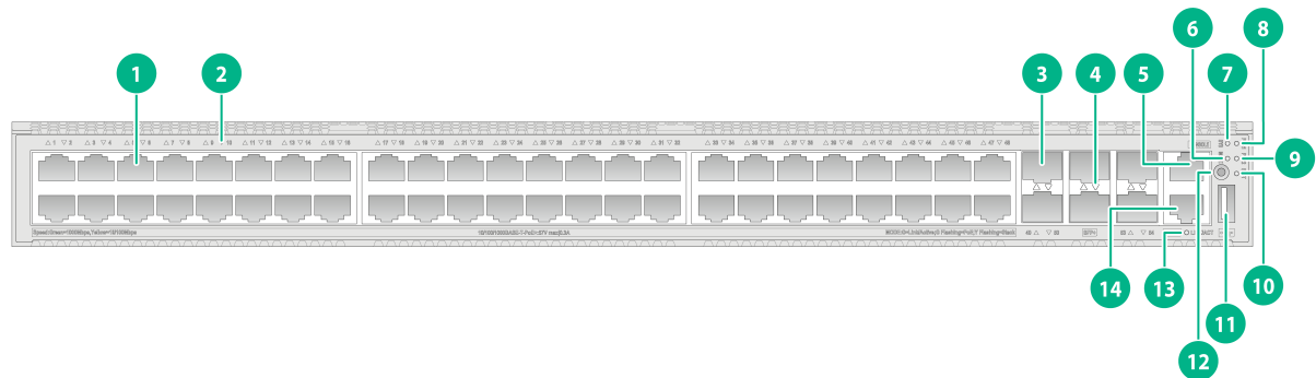
图2-6 S5800XP-56C-PWR-HI-G 前面板示意图
