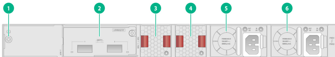
图2-8 PoE 机型后面板示意图
