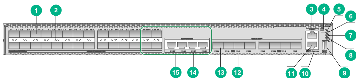
图2-2 S5800XP-40F-HI-G 前面板示意图
