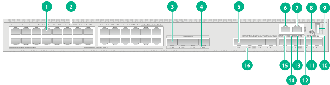
图2-5 S5800XP-38C-PWR-HI-G 前面板示意图
