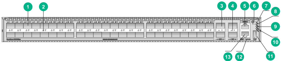
图2-4 S5800XP-56F-HI-G 前面板示意图
