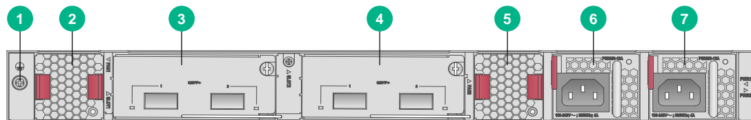
图2-7 非 PoE 机型后面板示意图
